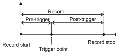
Image 0.47: Déclenchement dans l'enregistreur de forme d'onde
