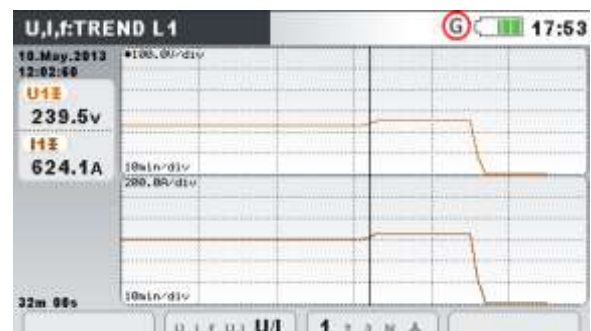
Image 0.19: Tendance de tension et de courant (mode double)
