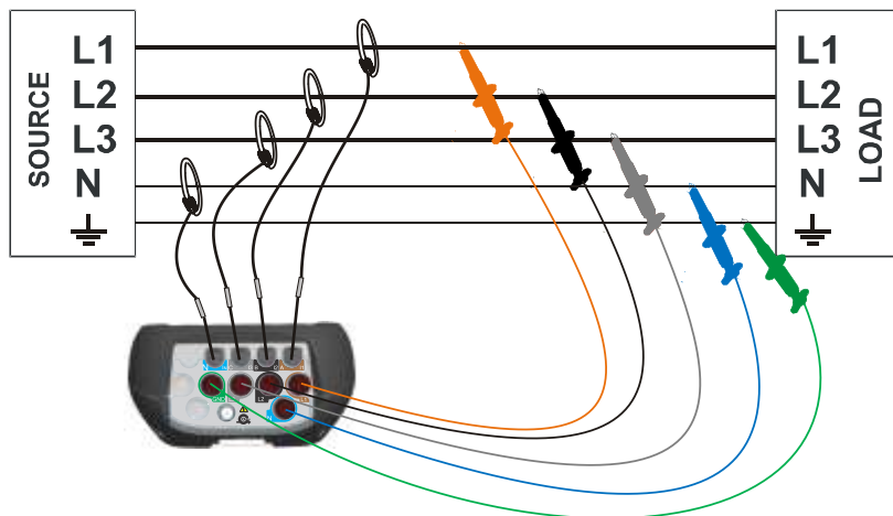
Image 0.4: Système triphasé à 4 fils
