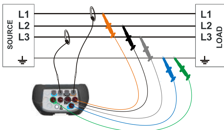
Image 0: Système Open Delta (Aaron) à 3 fils
