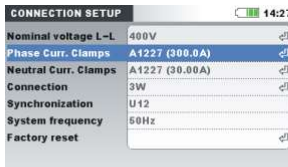
Image 0: Réglage de la reconnaissance automatique des pinces
