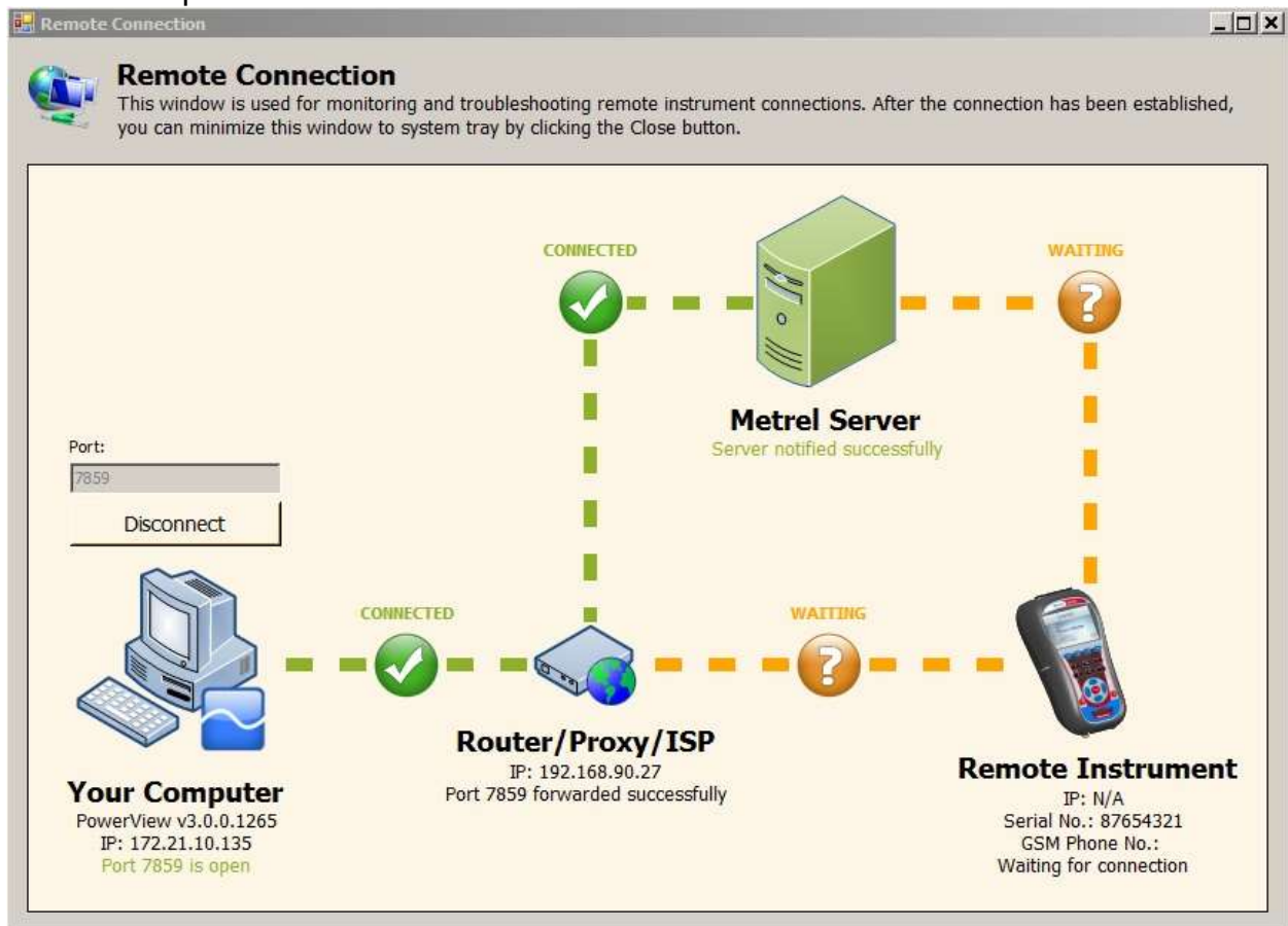
Image 0.12: Connexion PowerView au réseau local( LAN) et au serveur Metrel établie (Etapes 1 et 2)
