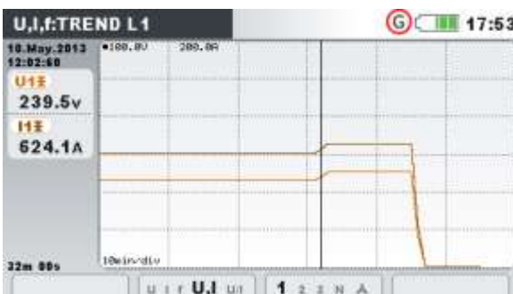
Image 0.18: Tendance de tension et de courant (mode unique)
