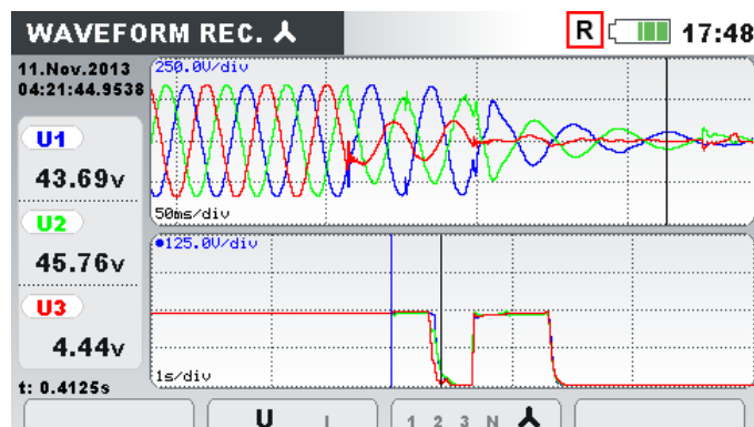
Image 0: Ecran de l'enregistreur des formes d'ondes enregistrées
