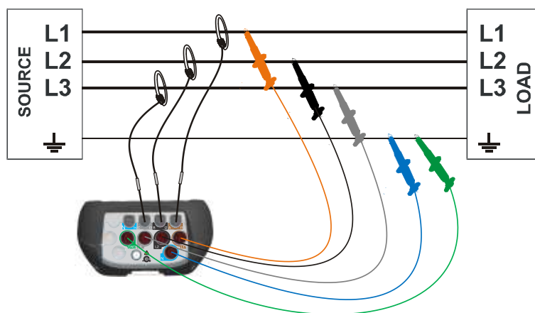
image 0.6: Système triphasé à 3 fils
