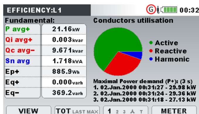
Figure 0.29: Ecran Efficacité Energétique
