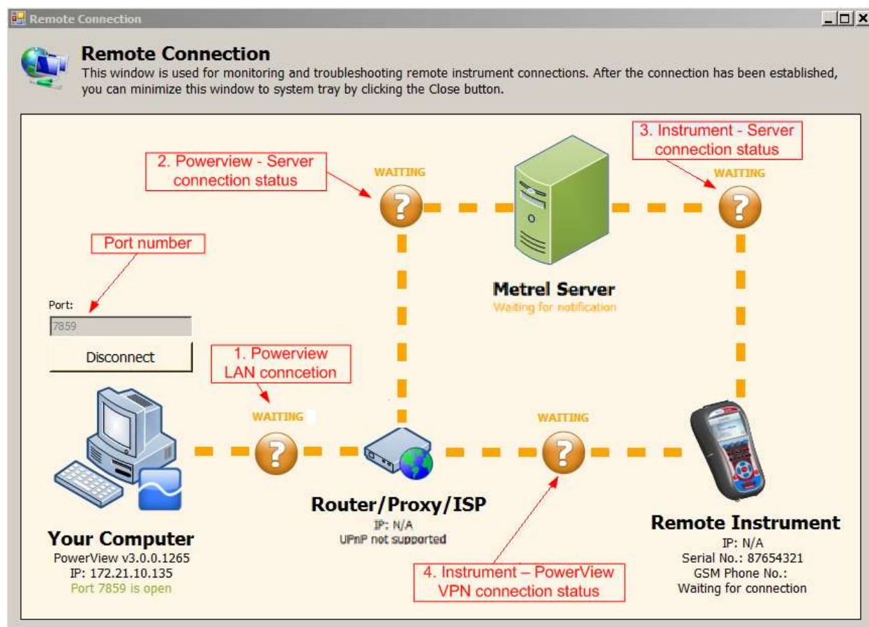
Image 0: Contrôle de connexion à distance PowerView v3.0
