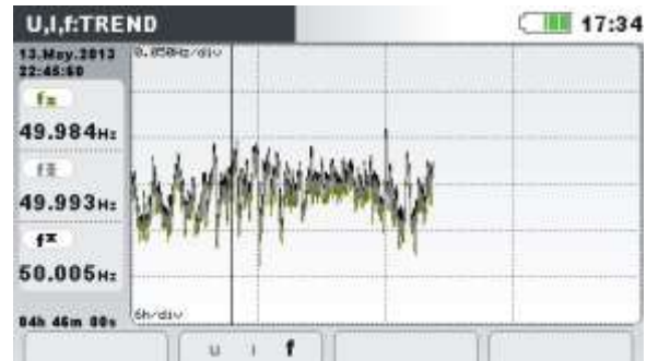
Image 0.21: Tendance de fréquence
