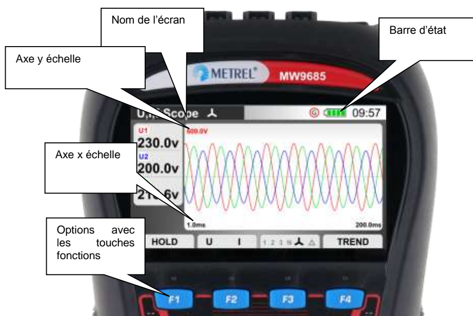
Image0.2: Affichage typique lors de mesure
