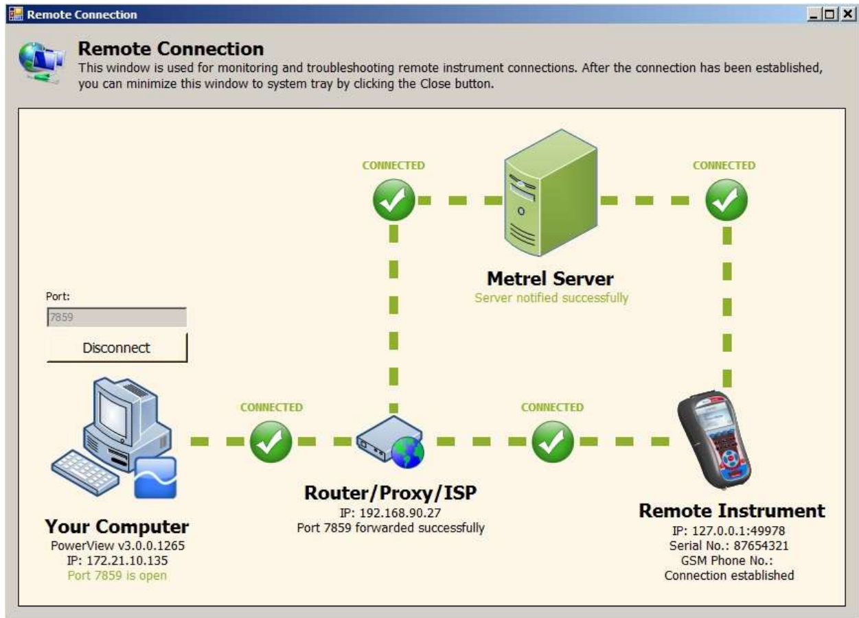
Image 0: Connexion à distance de l'appareil au PowerView v3.0 établie (Etape 4)
