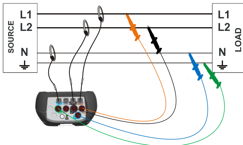
Figure 0.8: Système 2 phases 4 fils
