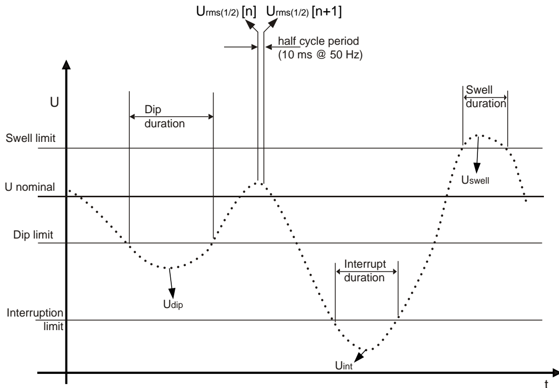
Image 0.9 Définition des évènements de tension
