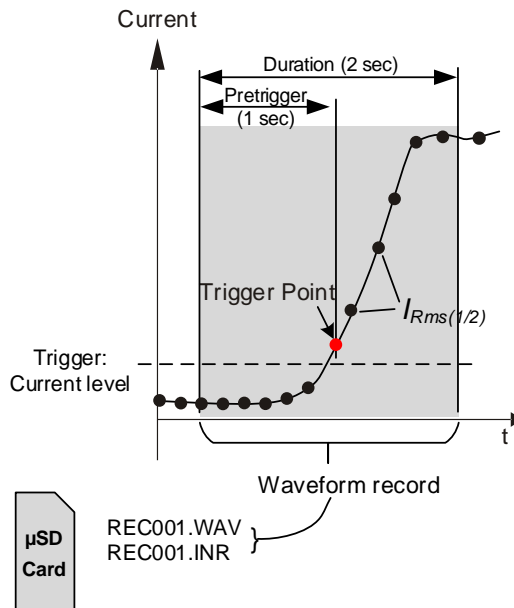
Figure 0.16: Déclenchement par niveau d'intensité (Inrush)
