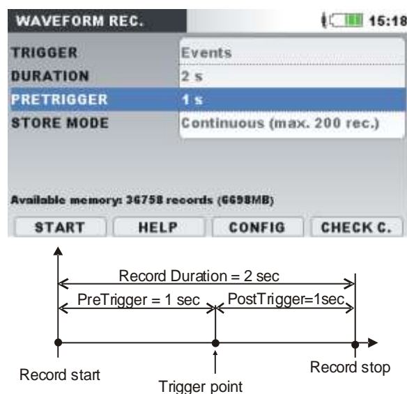
Figure 0.13: Description de déclenchement et de phase pré-déclenchement
