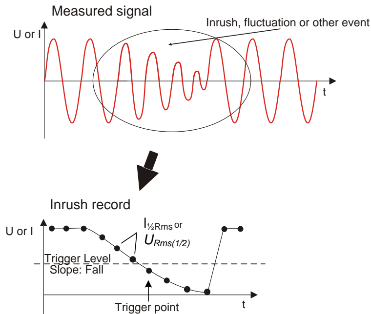
Image 0.13: Niveau de déclenchement
