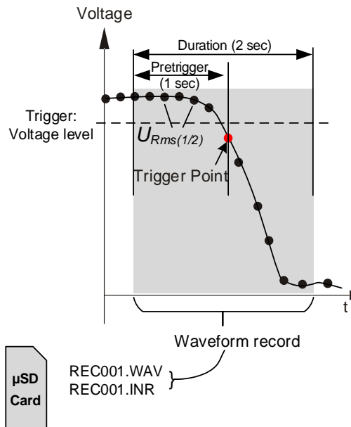
Figure 0.15: Déclenchement par niveau de tension
