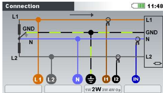
Figure 0.7: Sélection du système 2 phases 4 fils sur l'instrument
