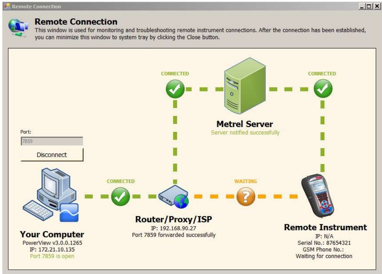
Image 0: Connexion à distance de l'appareil au serveur Metrel établie (Etape 3)
