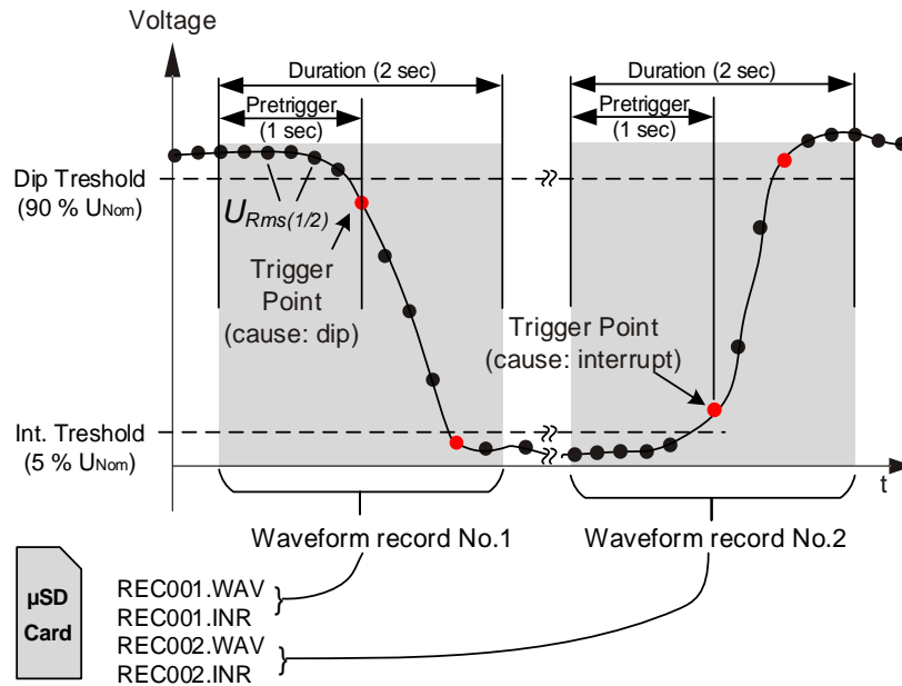
Figure 0.14: Déclenchement d'évènement de tension
