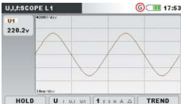
Image 0.12: Forme d'onde unique de tension
