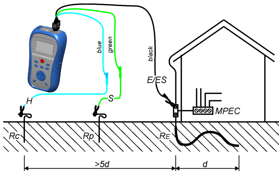
Schéma 4.33: Résistance de terre, mesure de la mise à la terre principale d'une installation
