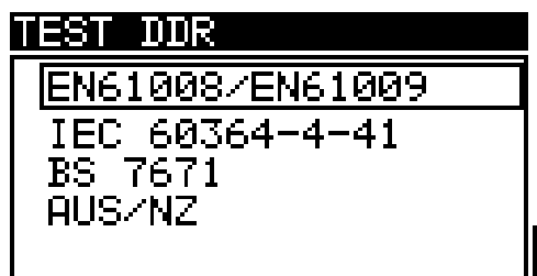
Figure 3.4: Sélection de norme pour test DDR
