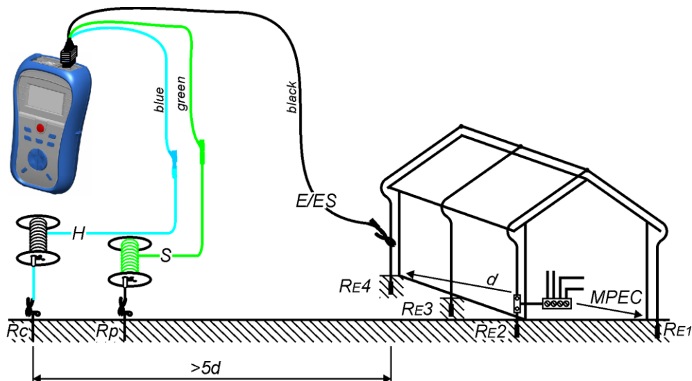
Figure 4.34: Résistance de terre, mesure sur un système de protection paratonnerre.
