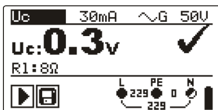
Schéma 4.18: Exemple de résultats de mesure de tension de contact
