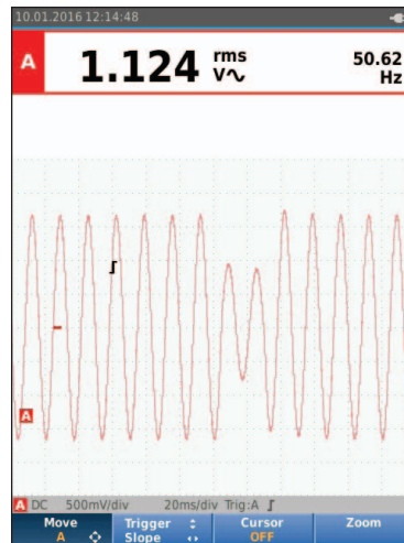
Le point de déclenchement est réglé sur un point, mais à cause de l'aberration du front ascendant au cours de la seconde période, un déclenchement supplémentaire déstabilise l'affichage.
