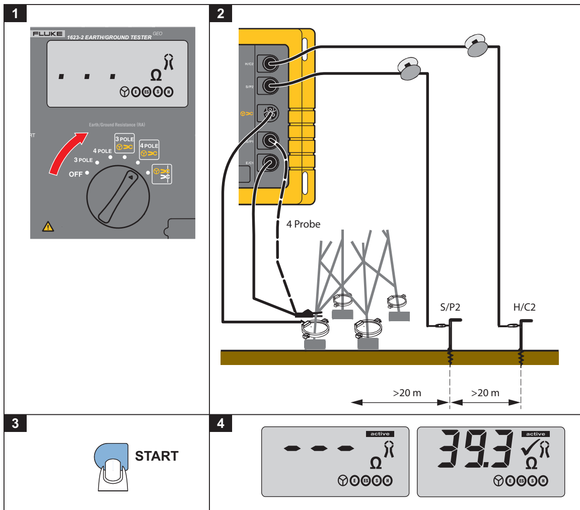
Figure 9. Résistance de mise à la terre sans débrancher le câble de garde
