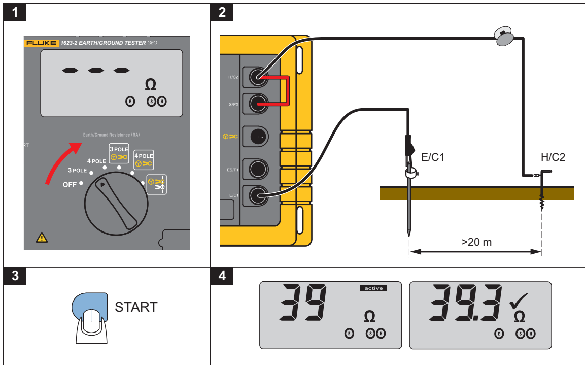
Figure 3. Mesure bipolaire R_A
