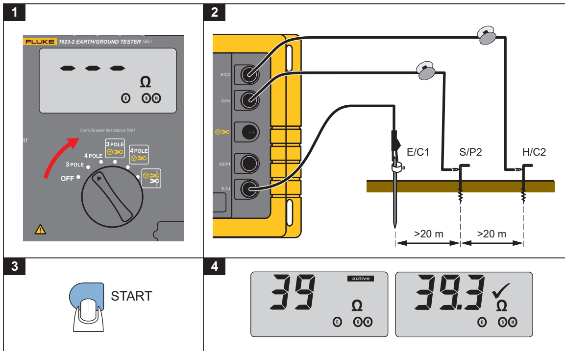
Figure 4. Mesure tripolaire R_A
