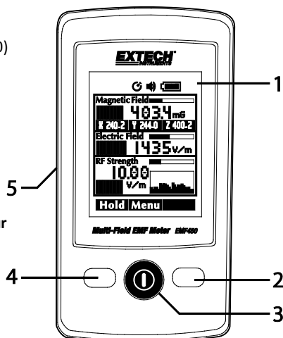
Figure 1 - Description du compteur
