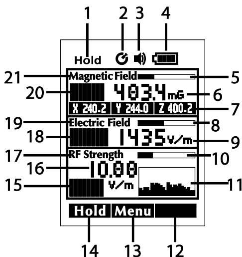
Figure 2 – Description de l'écran
