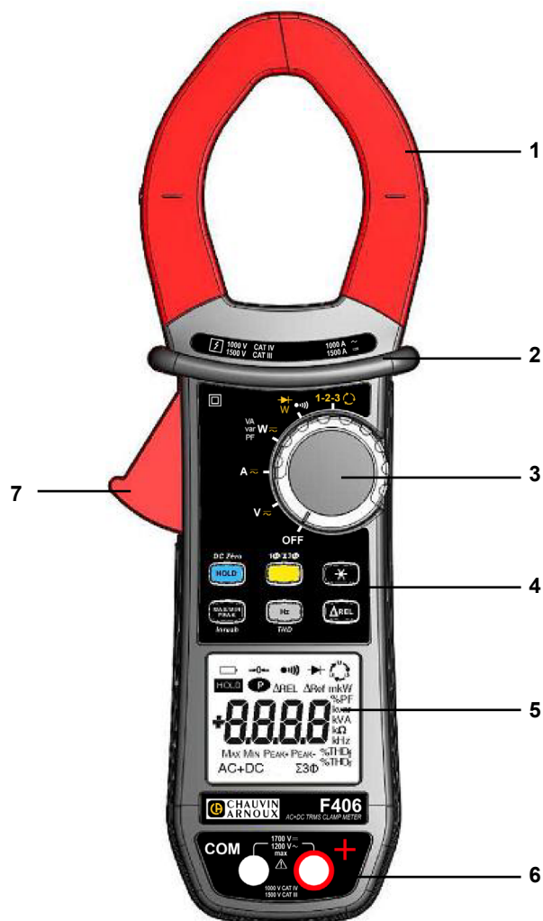
Figure 1 : la pince multimètre F406
