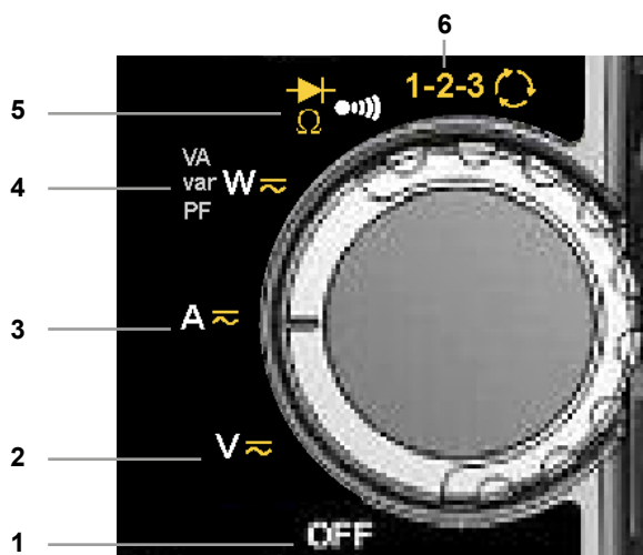
Figure 2 : Le commutateur
