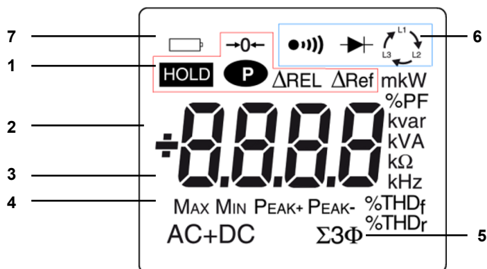
Figure 4 : L'afficheur
