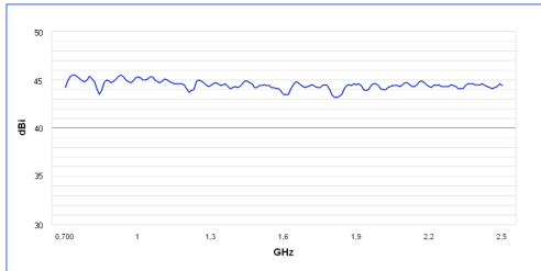
Diagramme de gain HyperLOG 7025X
