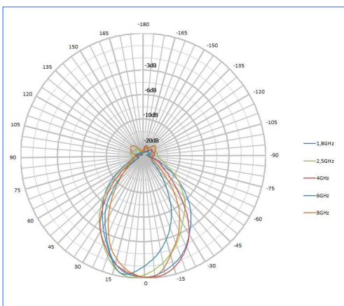
Modèle horizontal Série HyperLOG 60.. X
