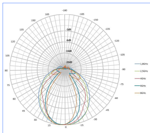
Modèle vertical Série HyperLOG 60.. X
