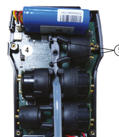
Cellule enlevée
