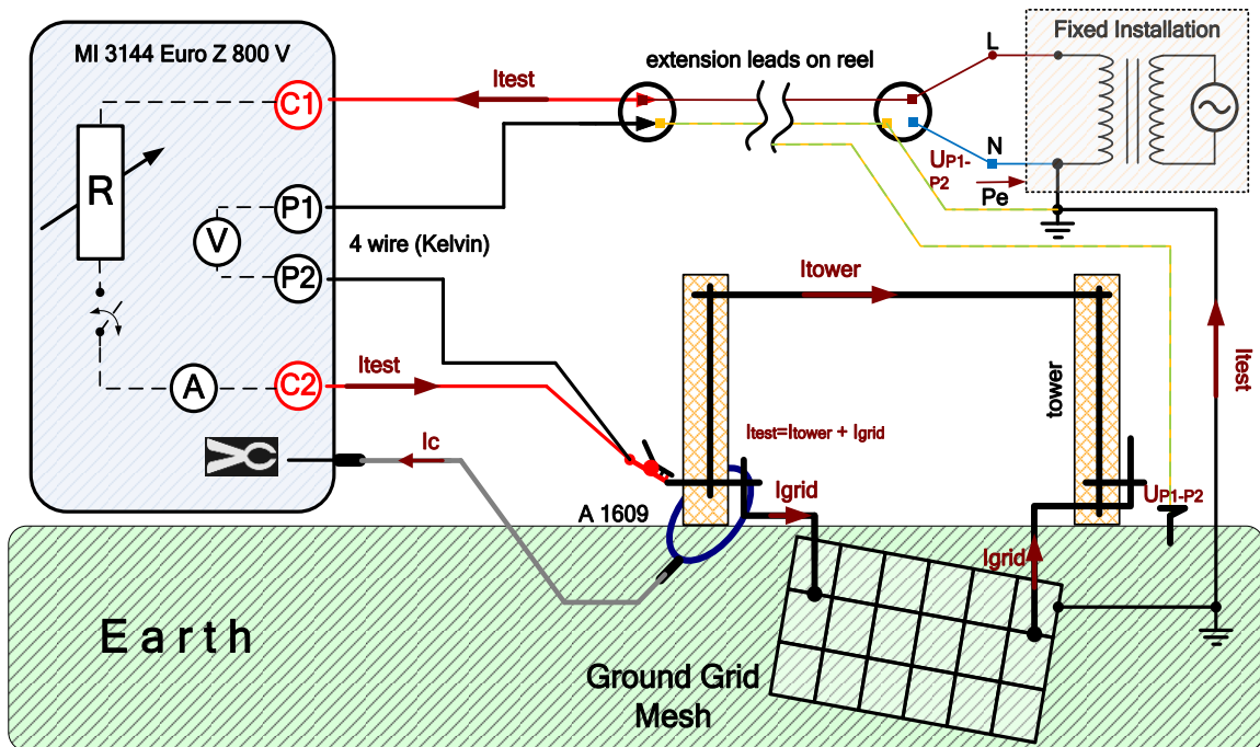
Image 6.6 : exemple 3 de mesure de courant élevée (IEEE-81)
