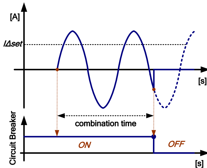
Image 6.20 : exemple de forme d'onde de courant de test DDR-M de temps de combinaison
