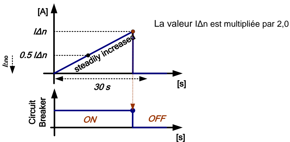
Image 0.3 : Exemple de formes d'ondes d'injection de courant de test (de type B)
