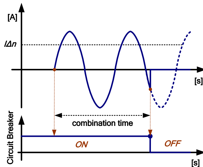
Image 0.4 : exemple de forme d'onde de courant de test DDR-M de temps de combinaison (de type AC)
