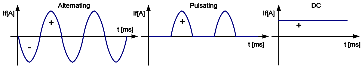
Image 9.2 : forme d'onde de courant
