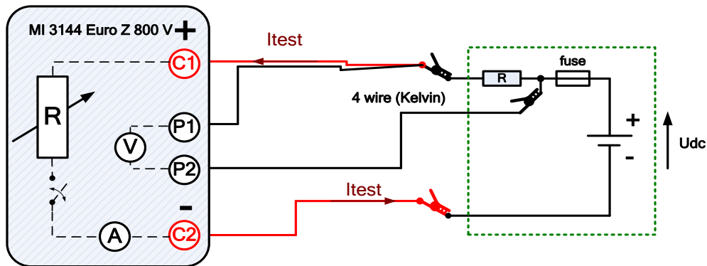
Image 6.11 : exemple 2 de mesure R line mΩ (installation DC)
