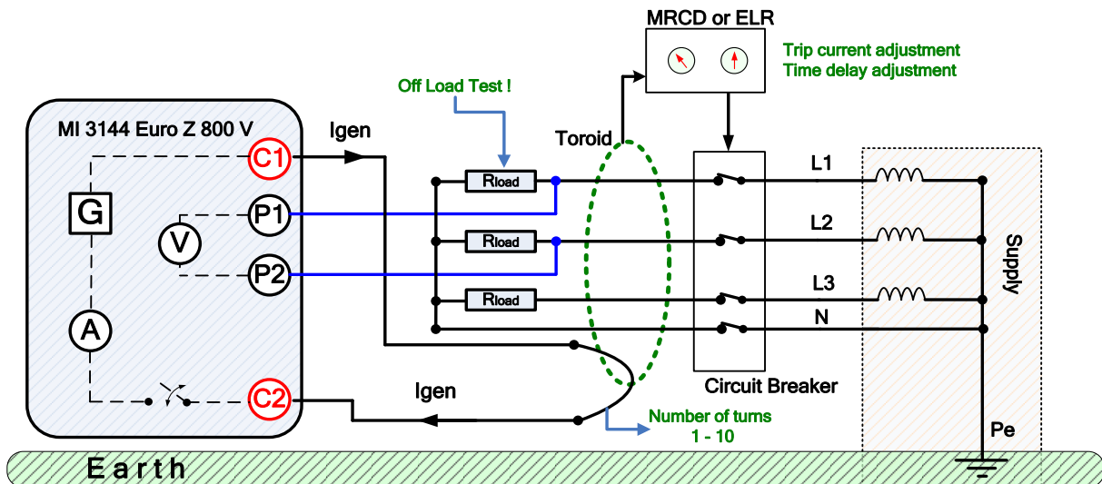
Image 6.16 : exemple de test DDR-M d'injection de courant et de temps de combinaison
