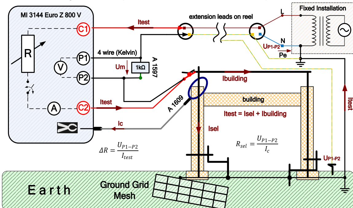
Image 6.7 : exemple 4 de mesure de courant élevé (IEEE-81)
