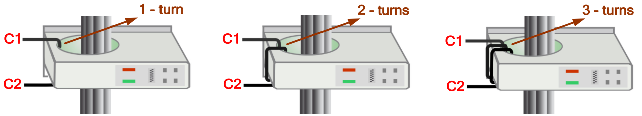
Image 6.19 : Nombre de tours - exemple
