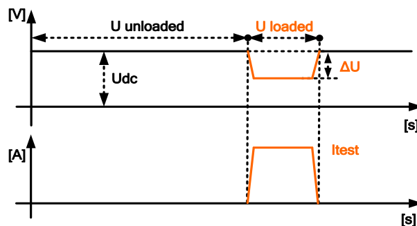
Image 6.12 : mesure R line mΩ - exemples de formes d'ondes de courant et de tension
