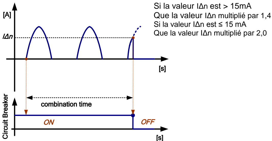
Image 0.5 : exemple de formes d'ondes de courant de test de temps de combinaison (de type A)
