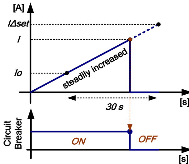
Image 6.18 : exemple de formes d'ondes du test d'injection de courant DDR-M
