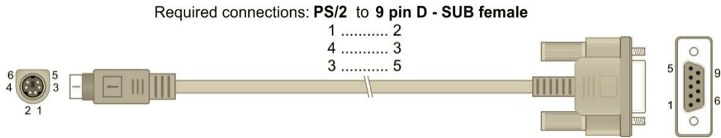
Image 7.1 : connexion RS-232 – (Exemple de connexion avec le MW9665)
