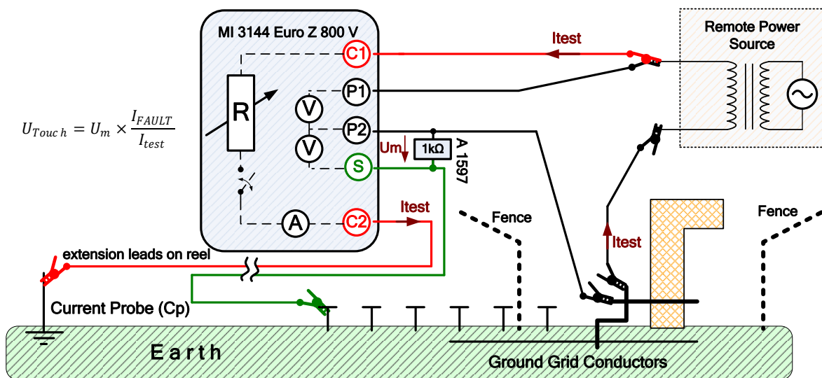
Image 6.14 : exemple de mesure U touch
