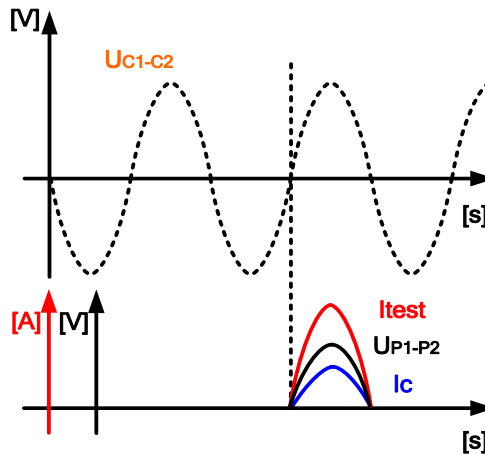
Image 6.8 : Exemples de formes d’ondes de courant et tension de mesure de courant élevée
