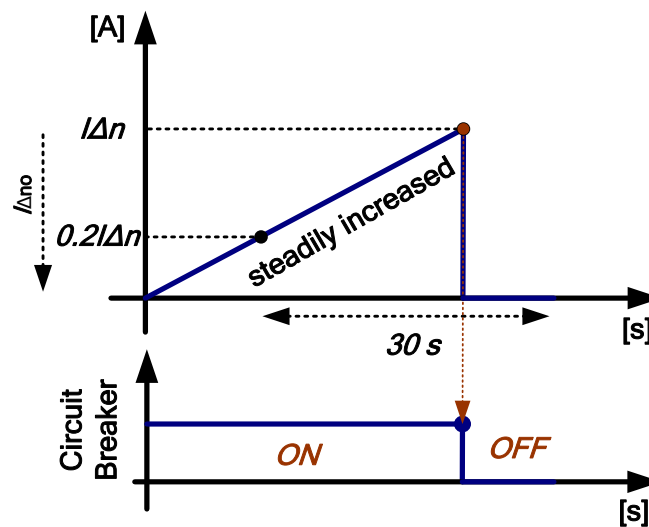
Image 0.1 : exemple de formes d'ondes d'injection de courant de test (de type AC)
