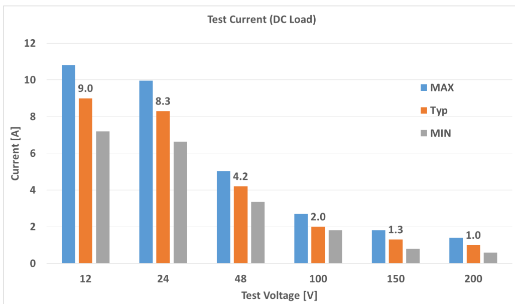
Image 9.1 : rapport entre le courant de test (charge de courant DC) et la tension nominale
