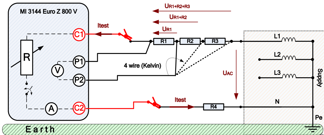
Image 6.4 : exemple 1 de mesure de courant élevé (panneau de distribution)
