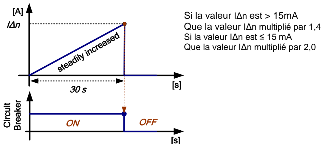
Image 0.2 : Exemple de formes d'ondes d'injection de courant de test (Type A)
