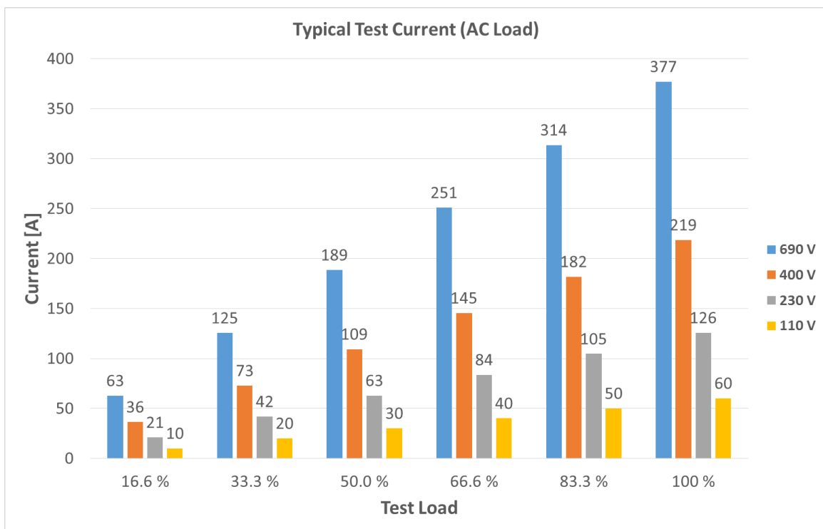
Image 9.3 : courants de test typique (charge AC) associés à la tension nominale et la charge de test
