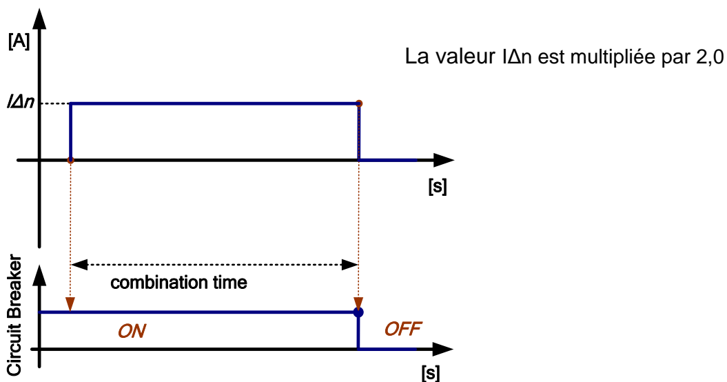
Image 0.6 : Exemple de formes d'ondes de courant de test de temps de combinaison (de type B)
