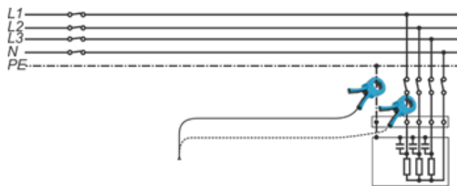
Image 6.22 : exemple de la pince A1281
