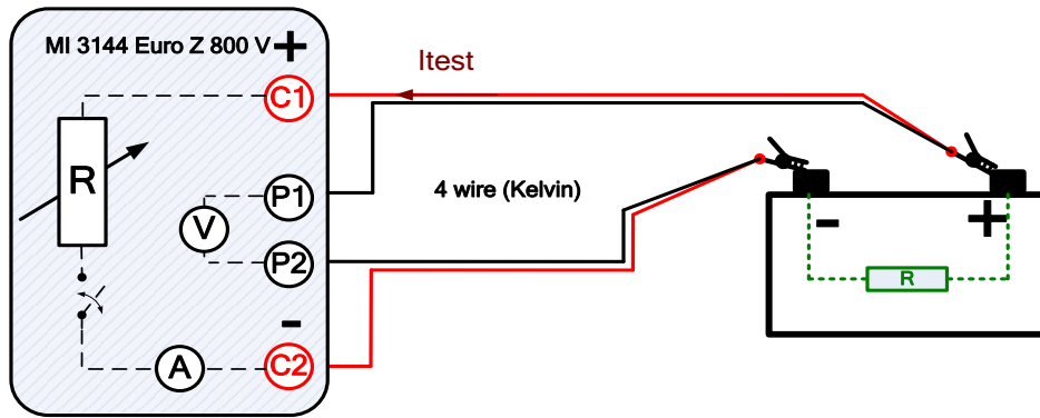
Image 6.10 : Exemple 1 de mesure R line mΩ (batterie)
