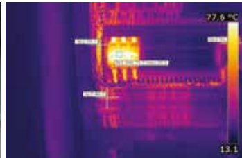
Les fusibles visibles sur l'image thermique sont surchargés et doivent être remplacés.
