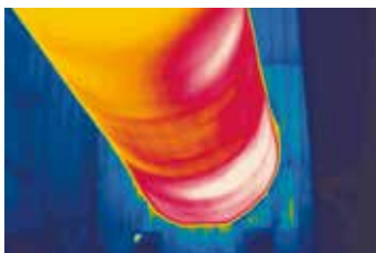
Détérioration du matériau réfractaire d'un four à ciment rotatif
