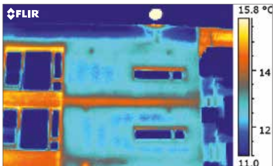
Pont thermique à l'un des étages.
