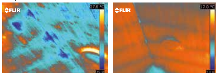
Deux images thermiques du même plafond. Sur l'image de gauche, l'humidité apparaît nettement car la pièce a été chauffée rapidement.
