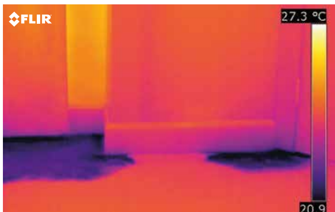
Diffusion d'humidité dans le sol, invisible à l'œil nu mais clairement visible sur l'image thermique.
