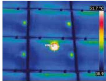
Ce point chaud dans une cellule photovoltaïque indique une détérioration physique interne.
