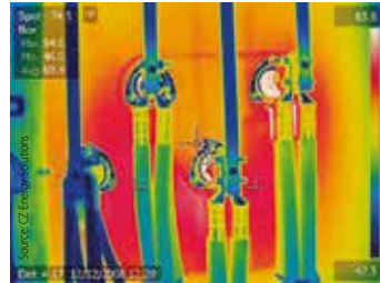
Les caméras thermiques permettent d'examiner tout le système d'installation, y compris les systèmes annexes de l'éolienne. Le connecteur de phase de droite est beaucoup plus chaud que les deux autres. Ce défaut a été identifié et réparé avant que la panne se produise.
