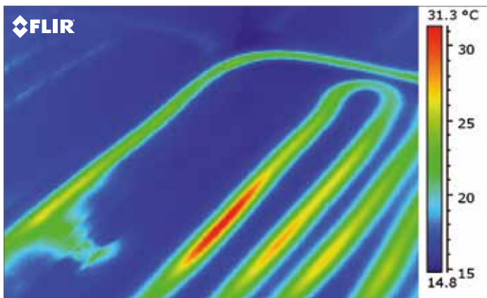
Fuite dans un système de chauffage par le sol.
