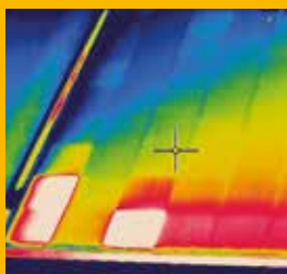
Cellules photovoltaïques défectueuses.
