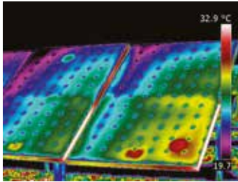
Ces points rouges signalent des modules nettement plus chauds que le reste, ce qui indique des connexions incorrectes.
