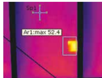
Cette image thermique montre un point chaud dû à une rupture de cellule dans un module standard de 60 cellules.
