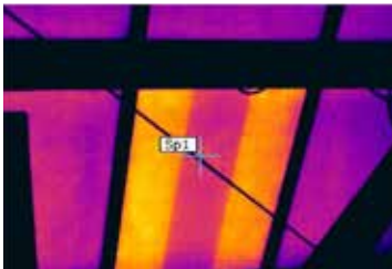
Deux séries de cellules apparaissent chaudes sur l'image thermique, ce qui indique une défaillance des diodes bypass.
