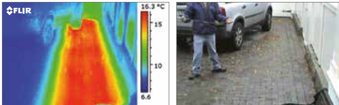
Une caméra thermique permet de localiser facilement les défaillances des systèmes de chauffage urbain.
