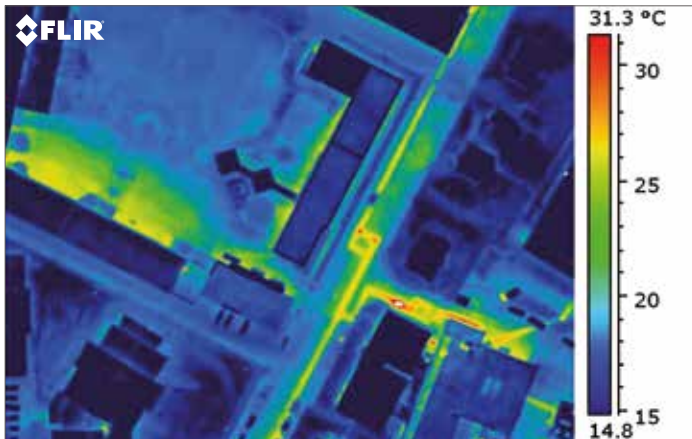
une image thermique prise à partir du haut identifie les fuites d'énergie dans un système de chauffage urbain.
