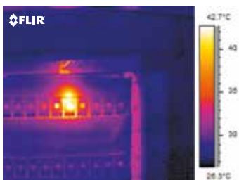
Surchauffe de l'un des fusibles, entraînant un risque d'incendie.
