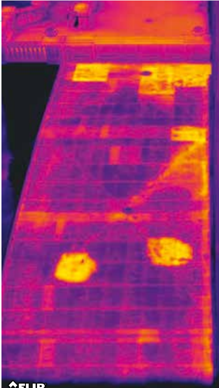
Humidité dans l'isolation d'un toit en terrasse.
