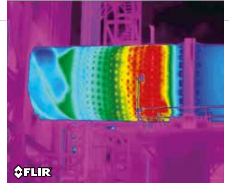
Four rotatif présentant une température de surface élevée.
