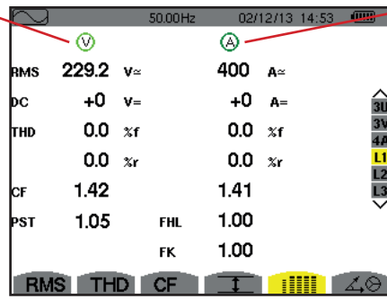
Figure 70 : L'écran affichage simultané en L1
