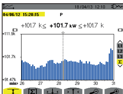
Figure 88 : P (Σ) avec MIN-AVG-MAX
