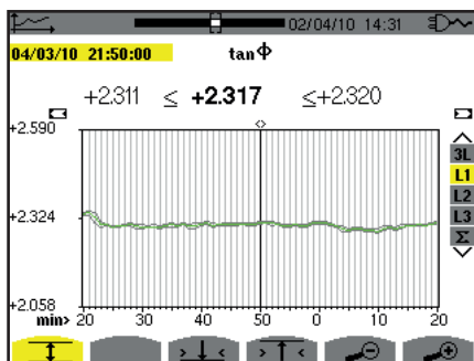
Figure 86 : tan Φ (L1) avec MIN-AVG-MAX
