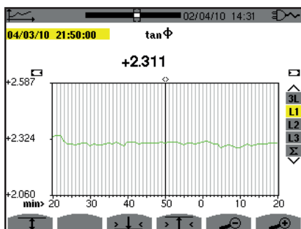
Figure 85 : tan Φ (L1) sans MIN-AVG-MAX pour un branchement triphasé avec neutre
