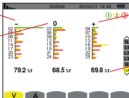
Figure 50 : L'écran du mode expert pour la tension simple (montages triphasés avec neutre)
