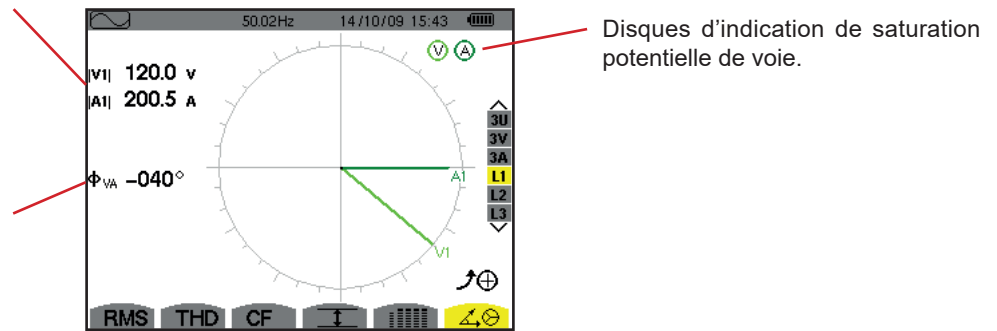
Figure 72 : L'écran d'affichage du diagramme de Fresnel en L1
